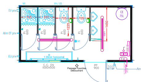
Configuration 3 : Bloc sanitaires REF ESSENTIEL EG5007HC / REF CONFORT EG500725 2 douches + 2 WC + 2 urinoirs + 1 auge
