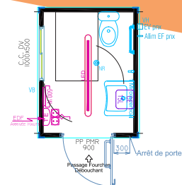
Configuration 2 : Bloc sanitaires PMR SPÉCIAL ÉVÈNEMENTIEL REF ESSENTIEL EG2002HC / REF CONFORT EG200225 1 WC + 1 lave-main
