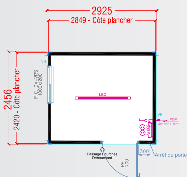
Configuration 1 : Usage polyvalent REF ESSENTIEL EG3005HC / REF CONFORT EG300525 1 fenêtre + 1 porte
