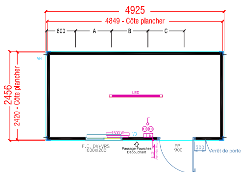
Configuration 1 : Usage polyvalent REF ESSENTIEL EG5008HC / REF CONFORT EG500825 1 fenêtre + 1 porte
