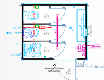
Configuration 3 : Bloc sanitaires REF ESSENTIEL EG3004HC / REF CONFORT EG300425 1 douche + 2 WC + 1 auge
