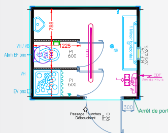
Configuration 2 : Bloc sanitaires REF ESSENTIEL EG3003HC / REF CONFORT EG300325 1 douche + 1 WC + 1 urinoir + 1 auge
