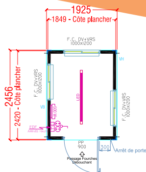
Configuration 1 : Guérite REF ESSENTIEL EG2001HC / REF CONFORT EG200125 3 fenêtres + 1 porte
