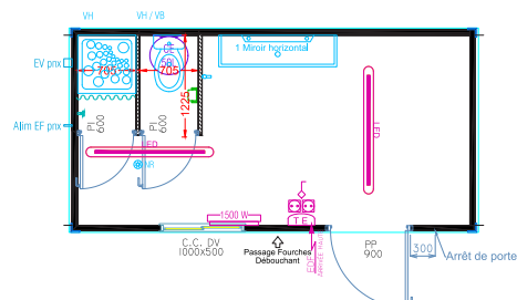
Configuration 2 : Sanitaires - Vestiaires REF ESSENTIEL EG5006HC / REF CONFORT EG500625 1 douche + 1 WC + 1 auge
